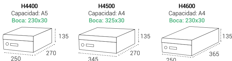
H4400-G3 Fondo 270 H4500-G3 Fondo 270 H4600-G3 Fondo 365
