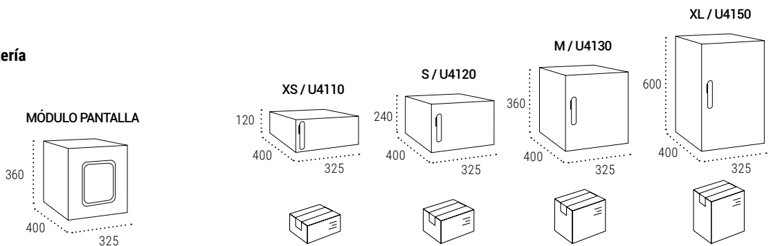
Agrupación de buzones de paquetería UNVERS DISPLAY para instalación a pared
