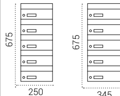
H4400-G5 Fondo 270 H4500-G5 Fondo 270 H4600-G5 Fondo 365
